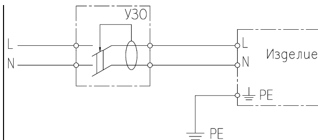
Рисунок 6б - Схема принципиальная подключения УЗО (GM-122/2,2)
