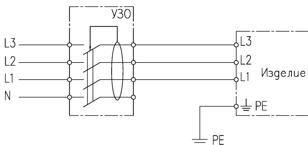
Рисунок 6а - Схема принципиальная подключения УЗО (GM-122/4,0)
